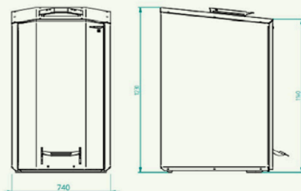
Abri-Bac 240 Litres
