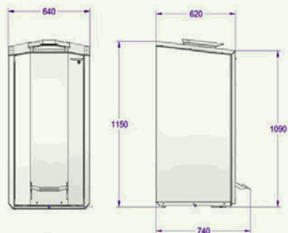
Abri-Bac 120 Litres
